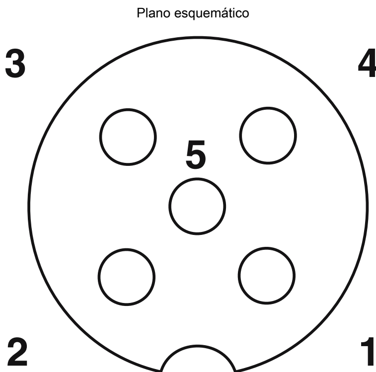
Esquema de polos del conector hembra M12, 5 polos, codificado A, vista de la cara de hembras
