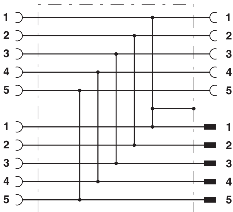
Ocupación de contactos del distribuidor H M12
