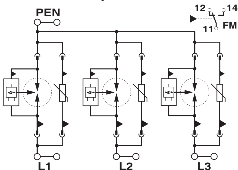
Diagrama eléctrico
