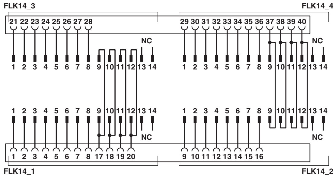
Anschlussbild FLKM 4X14-PA/AN/S7-1500
