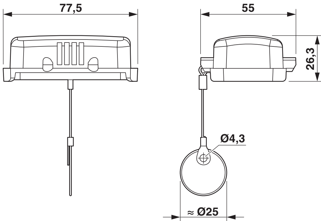
Maßzeichnung
