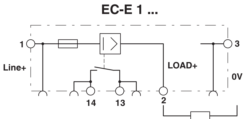
Diagrama eléctrico
