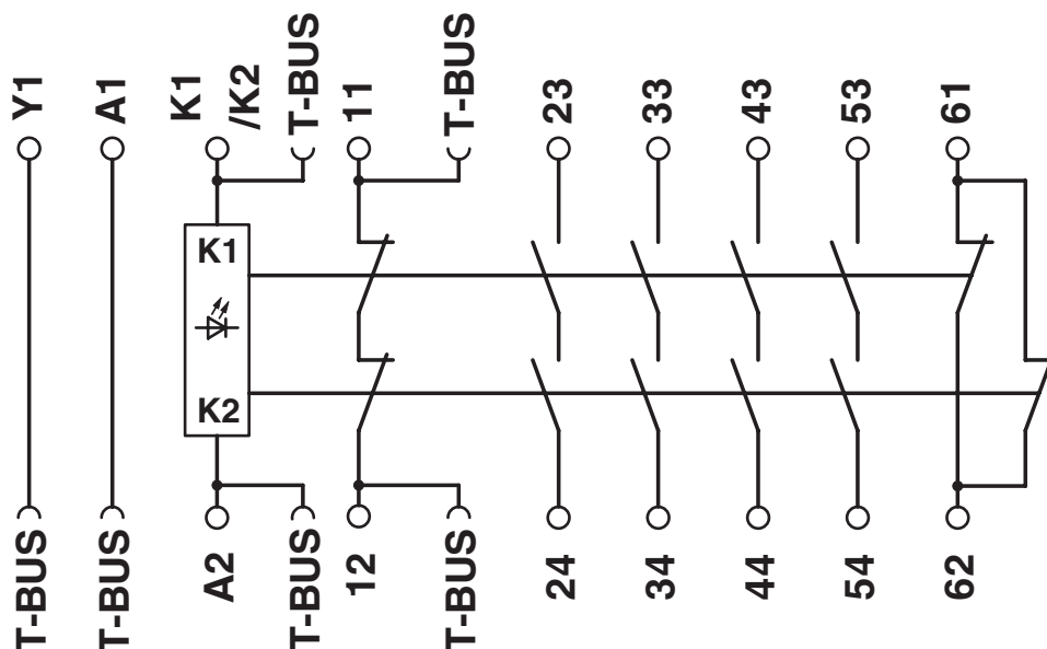
Diagrama eléctrico
