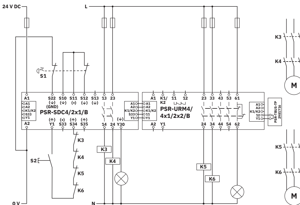
Control de parada de emergencia de dos canales con ampliación de contactos
