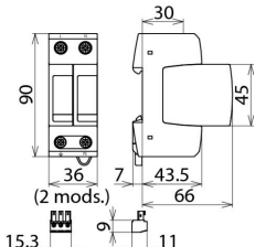
Dimensiones del DG MP TT 2P 275 FM
