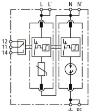
Esquema del DG MP TT 2P 275 FM
