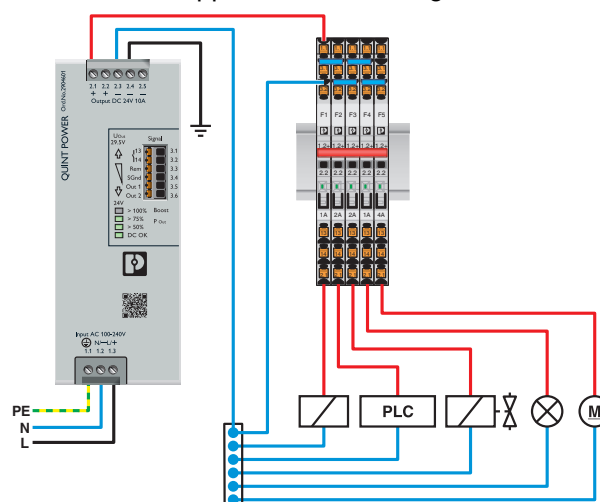
Applikationszeichnung
