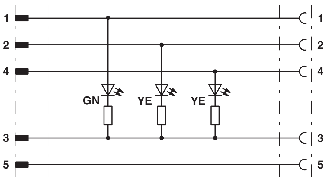
Ocupación de contactos de los conectores macho / hembra M12 con 3 LED
