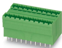
La figura muestra una variante de 10 polos con 20 contactos
