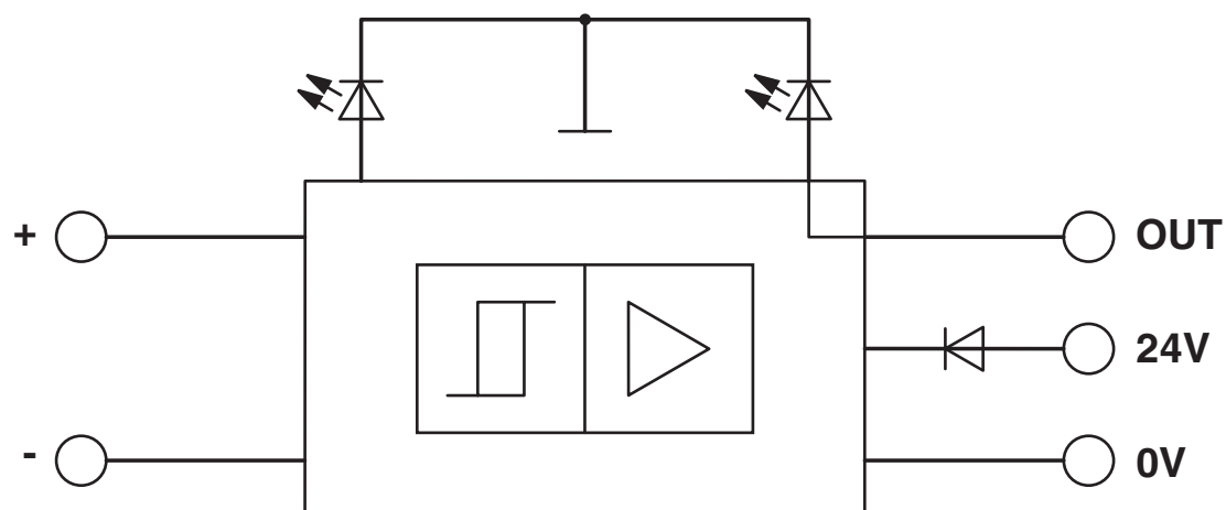
Schaltplan
