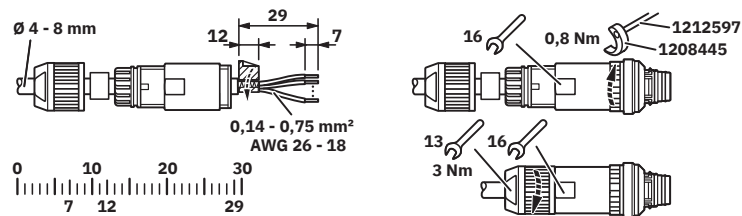
Dibujo funcional
