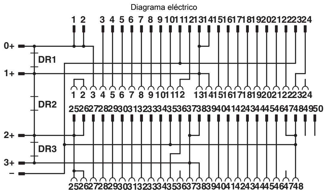
Esquema de conexiones FLKM 50-PA-S400
