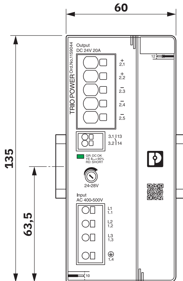
Maßzeichnung
