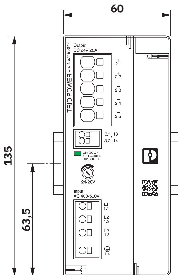
Dessin coté
