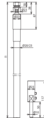
Maßbild HVI RAV 75 20 L6M SW M
