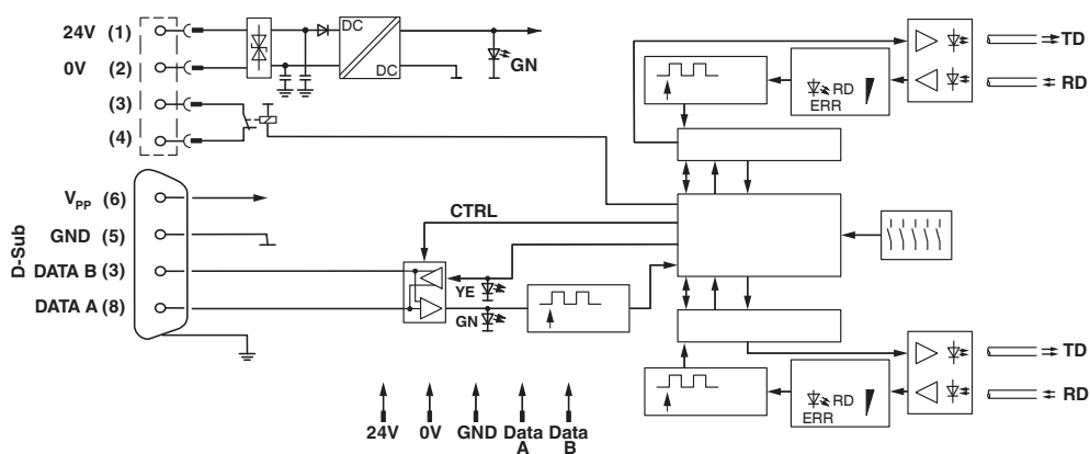
Blockschaltbild
