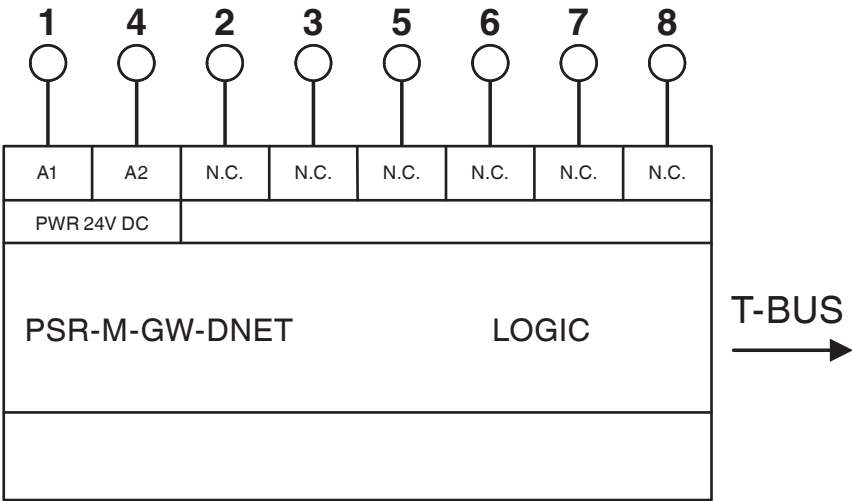
Blockschaltbild
