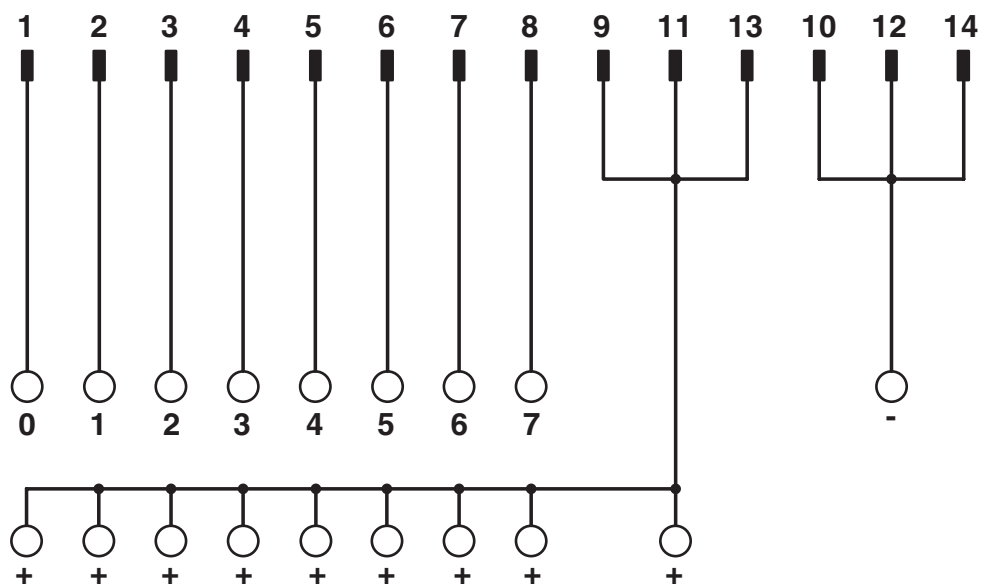
Diagrama eléctrico
