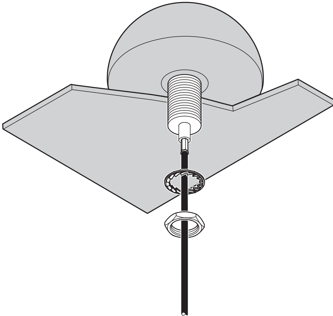
Schemazeichnung
