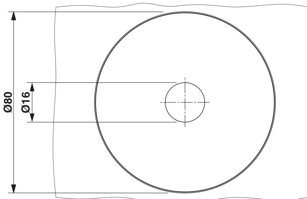
Maßzeichnung
