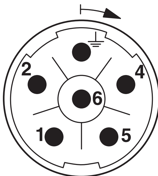
Plano esquemático
