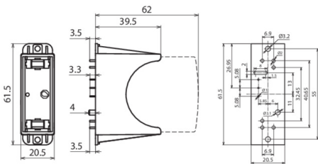
Dimensiones del DG PCB PV I 500 FM
