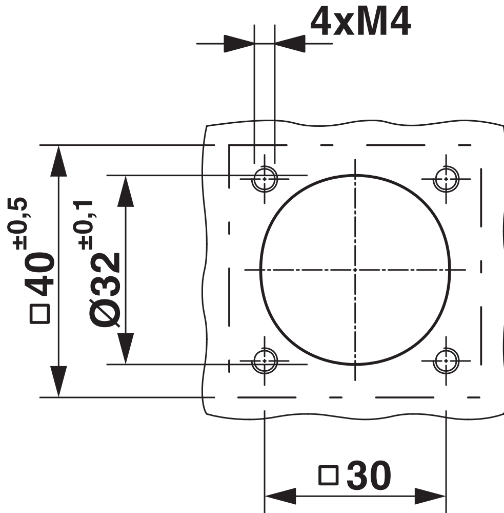
Maßzeichnung
