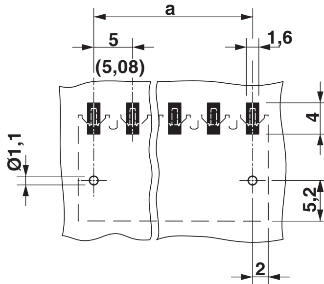
Bohrplan/Lötpadgeometrie
