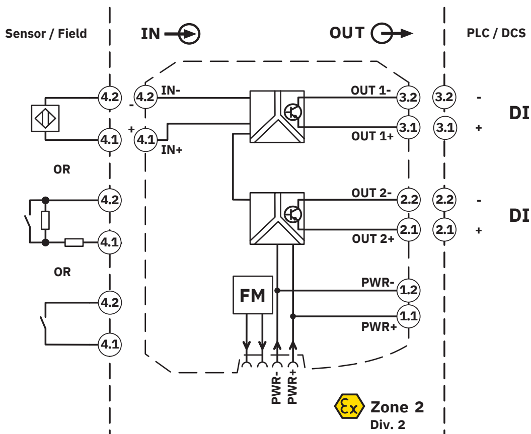
Schéma fonctionnel
