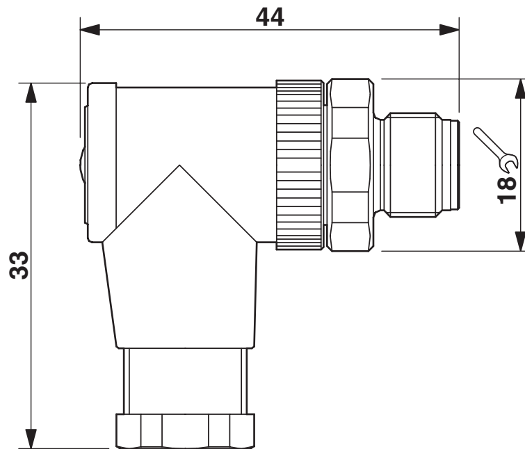
Maßzeichnung
