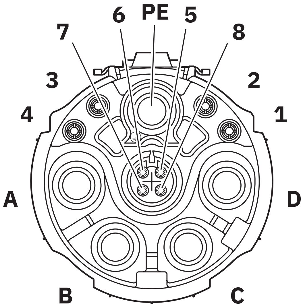
Polbild Buchse Signal, Kodierung 1
