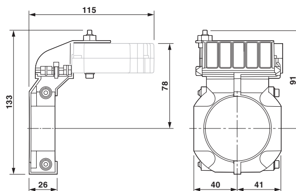
Ventilateurs pour la mise en place horizontale sur la traversée de paroi
