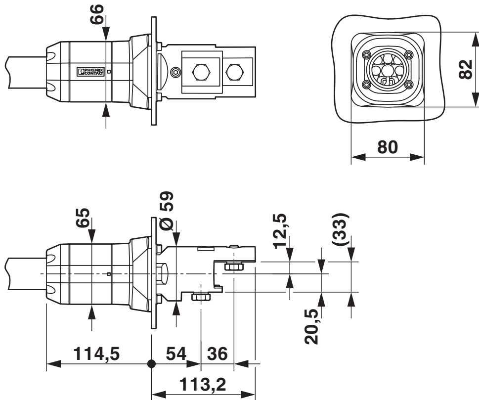
Dessin coté
