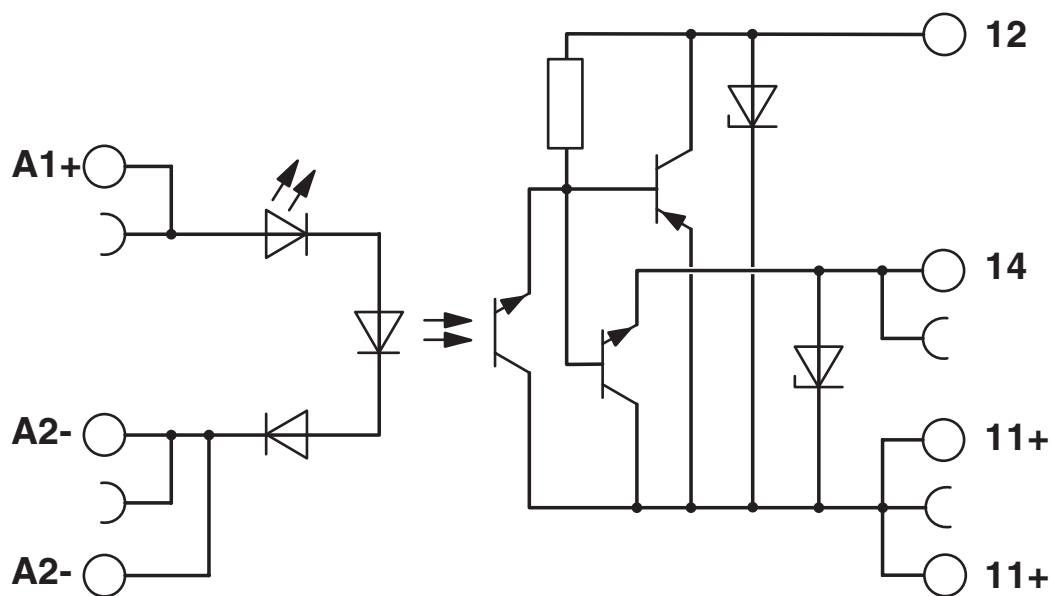
Diagrama eléctrico
