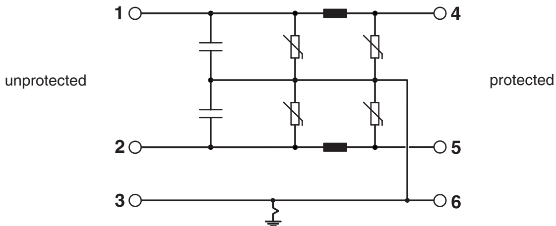
Schaltplan
