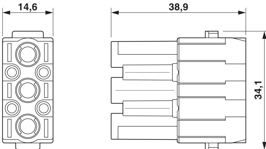
Maßzeichnung
