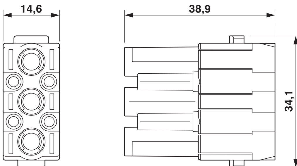
Dessin coté
