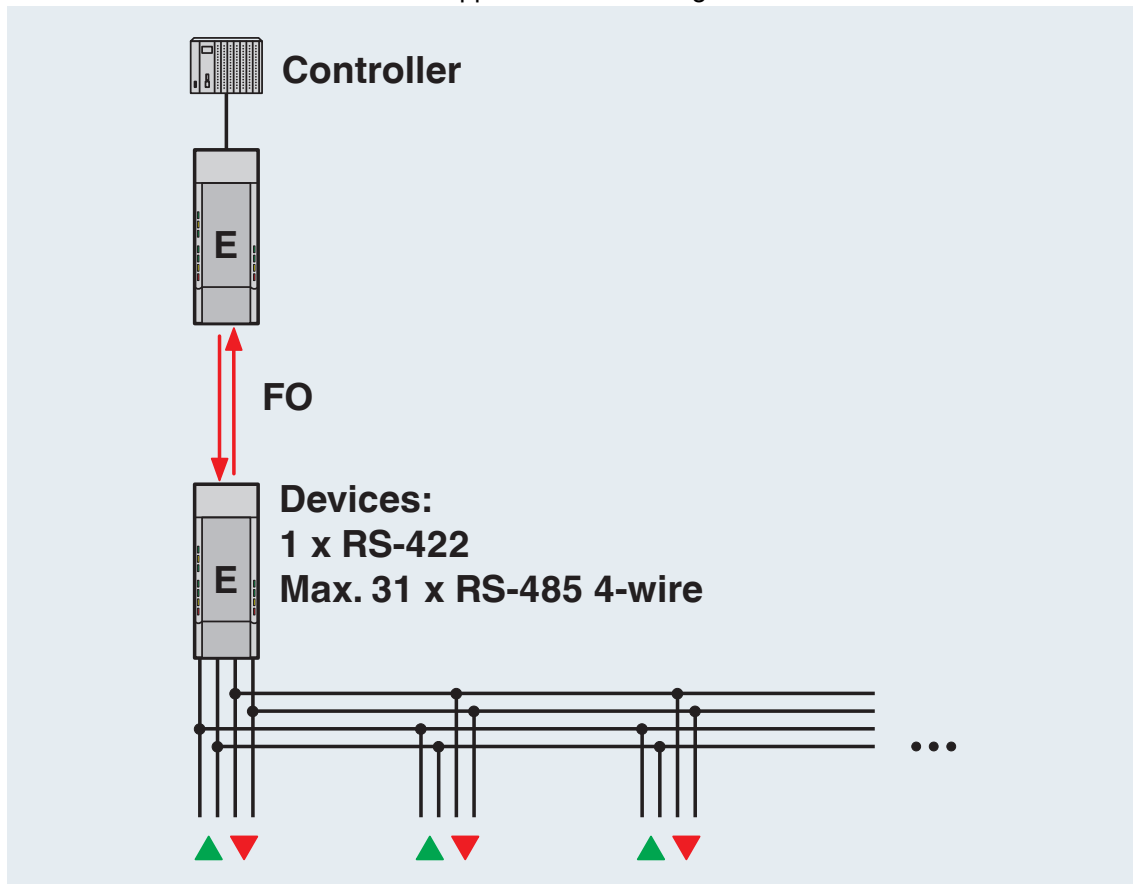
Punkt-zu-Punkt-Verbindung
