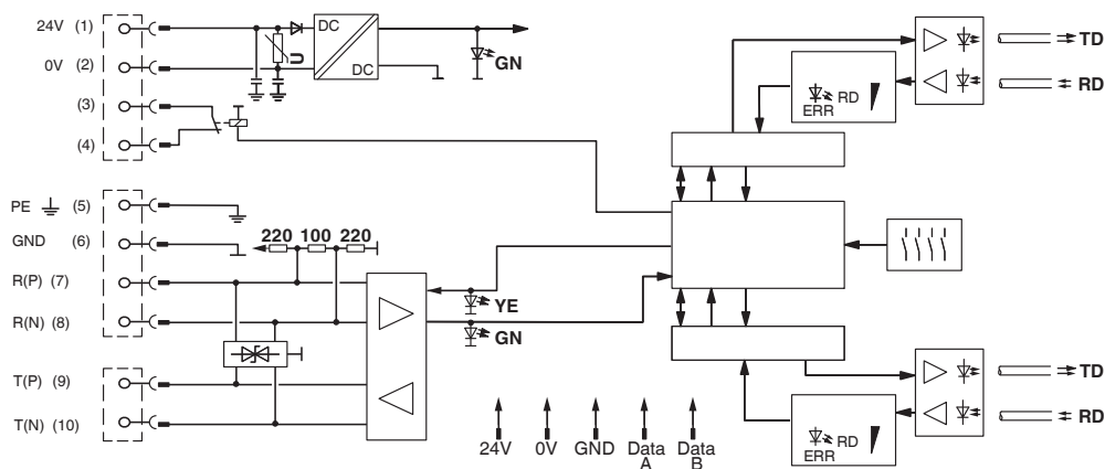
Schéma fonctionnel
