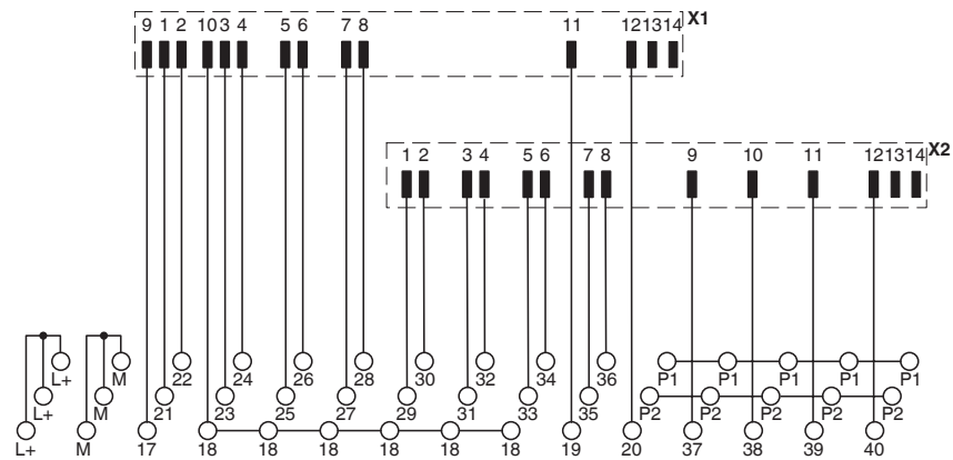
Schaltplan
