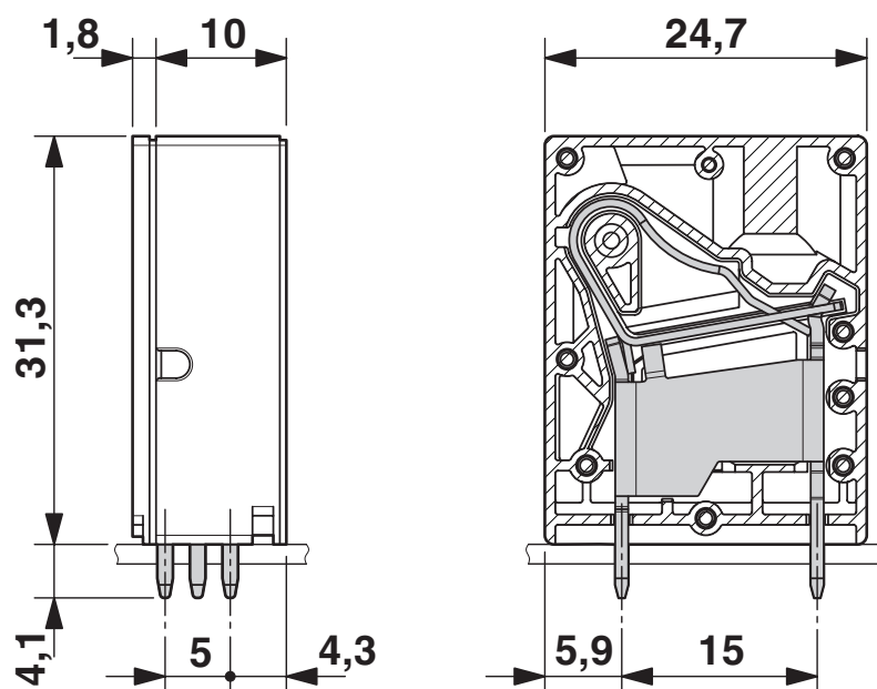
Maßzeichnung
