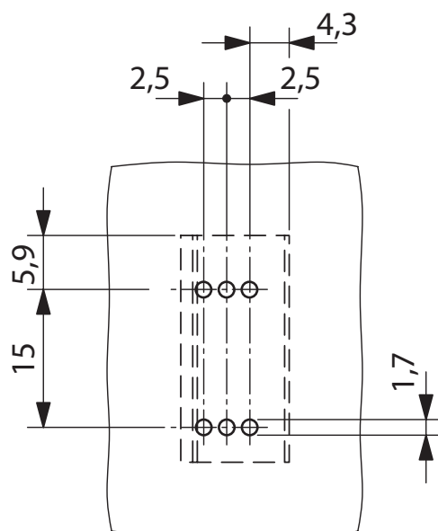
Bohrplan/Lötpadgeometrie
