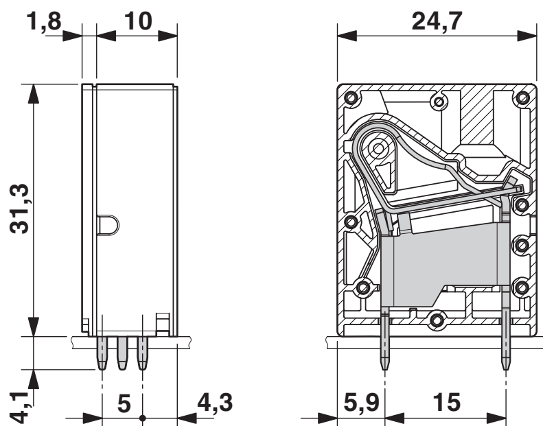
Dessin coté
