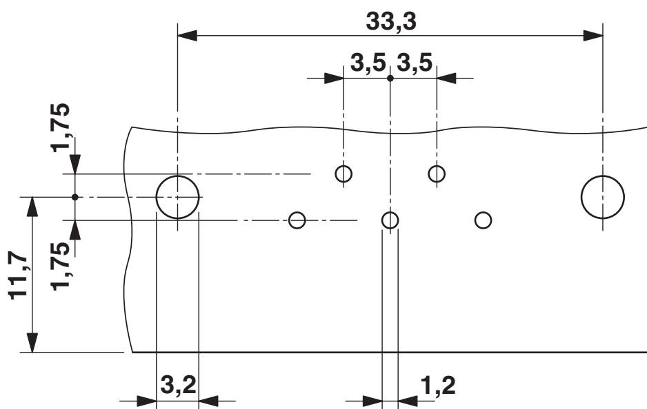
Esquema de taladros/geometría pads soldadura
