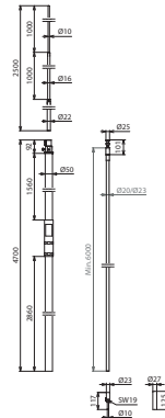
Maßbild HVI 20 M L6M SR4700 IP RFS2500
