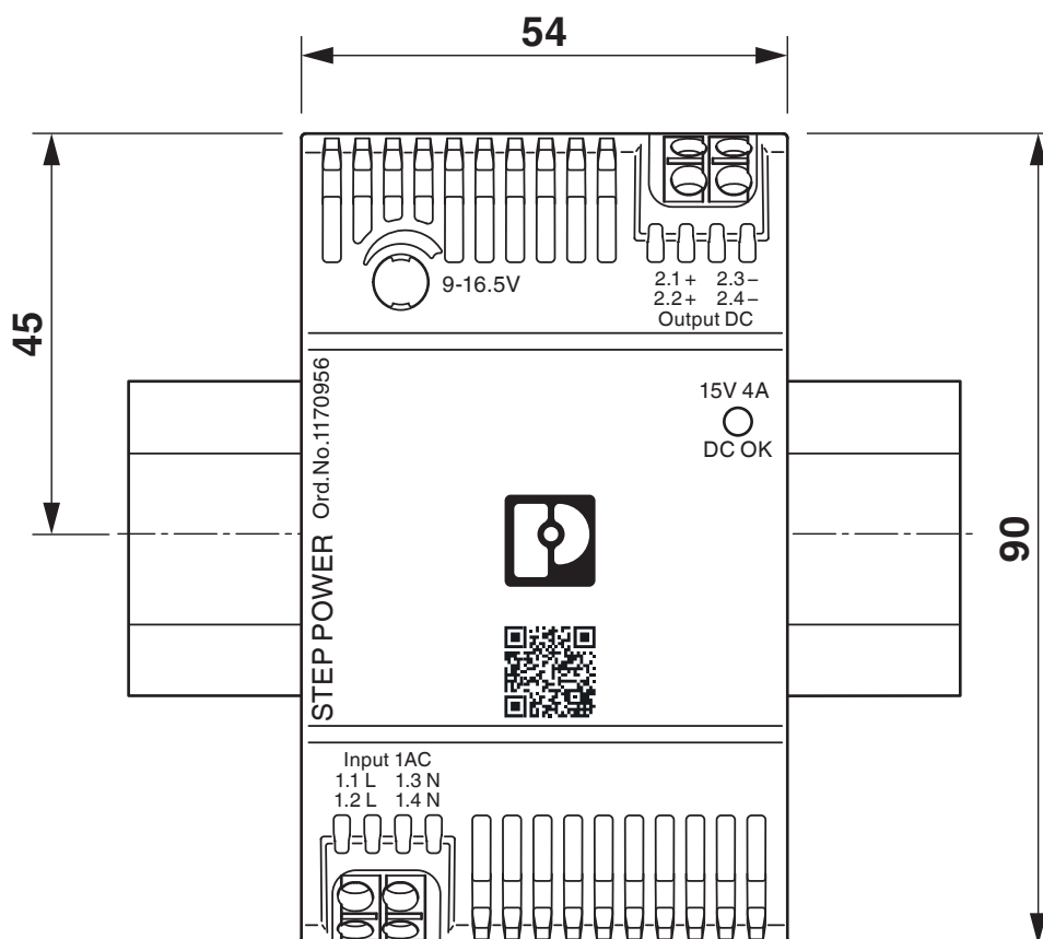
Maßzeichnung
