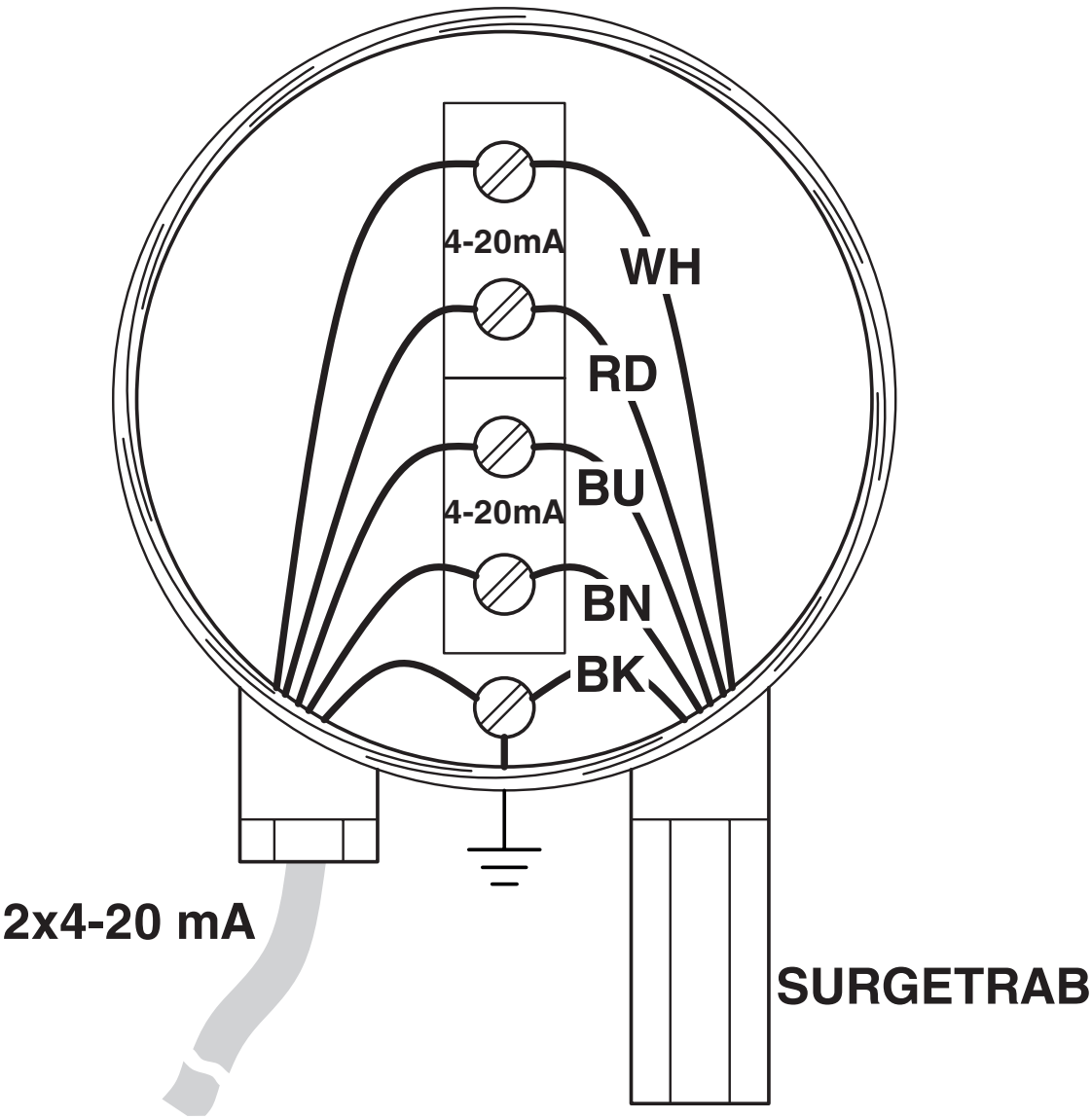
Applikationszeichnung
