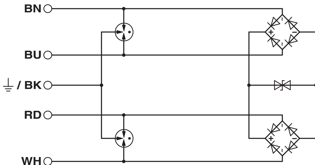
Diagrama eléctrico
