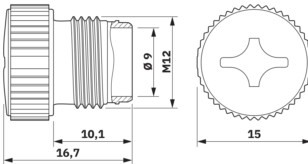
Dessin coté
