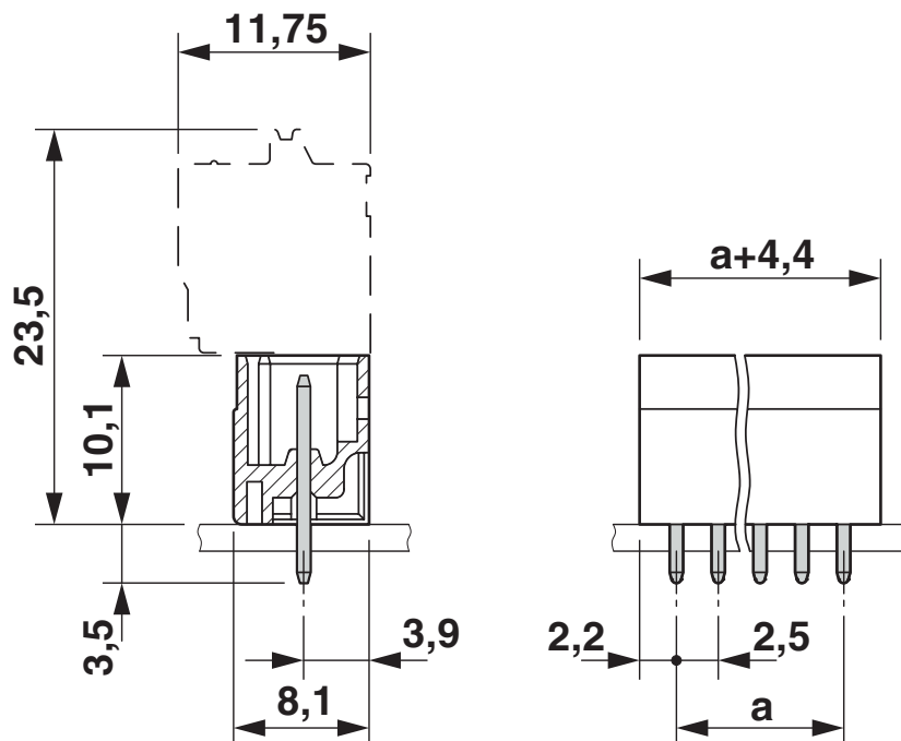
Dessin coté
