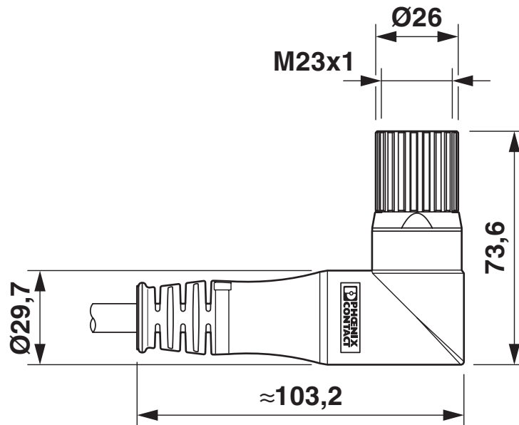
Maßzeichnung
