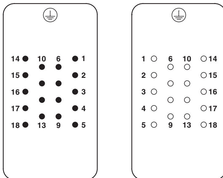
Plano esquemático
