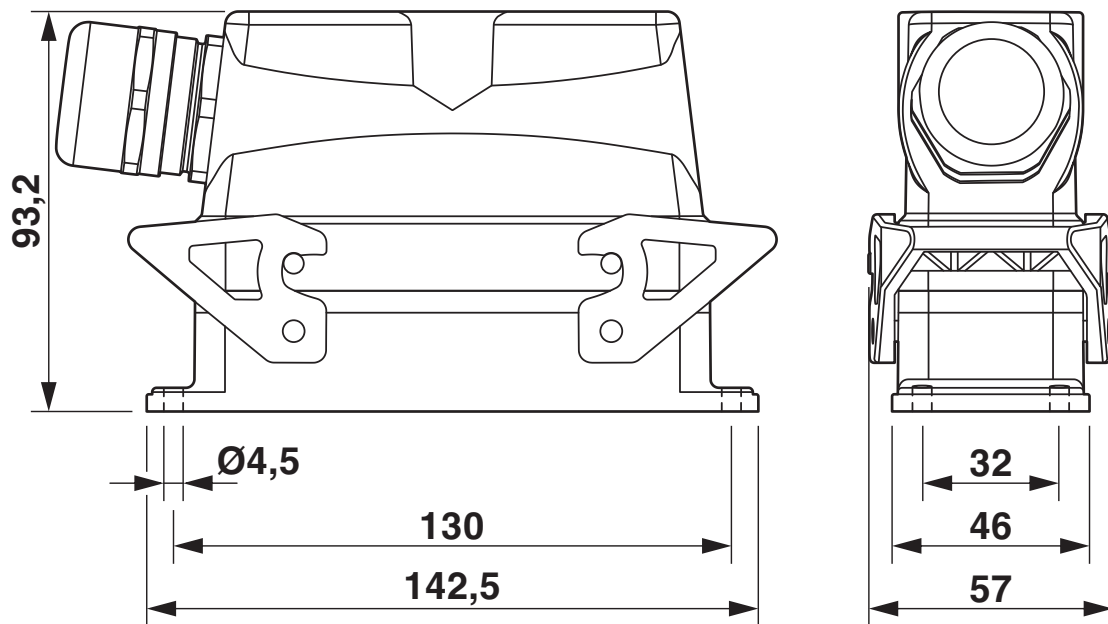
Maßzeichnung
