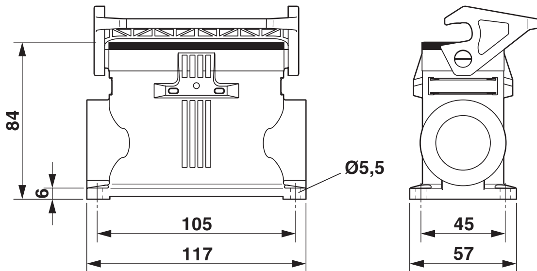
Maßzeichnung
