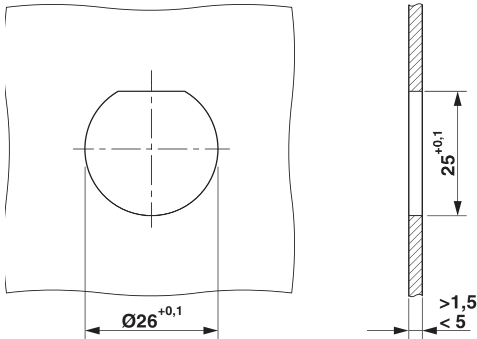
Maßzeichnung
