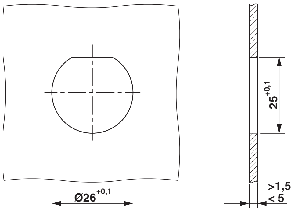
Dimensiones de montaje
